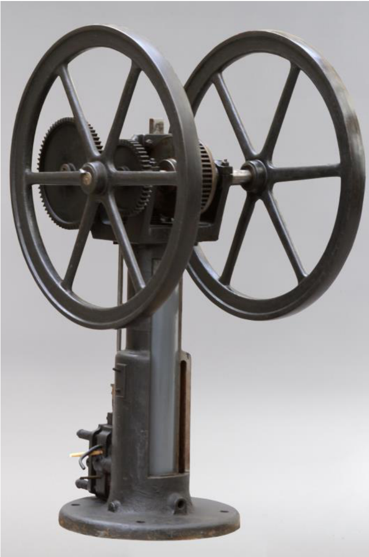
Stehender atmosphärischer Motor mit Flugkolben. (wie 731). Zu Lehrzwecken wurde der Zylinder geschnitten
