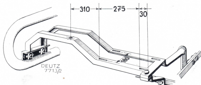
Anbringung des Fundamentrahmens am Binder
